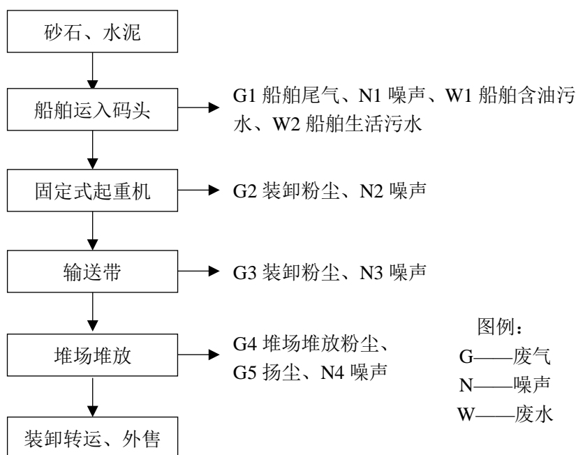
图 4-1 项目工艺流程及产污节点图
