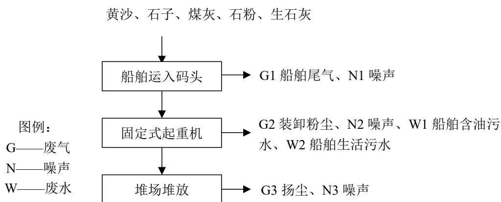
图 4-1 项目工艺流程及产污节点图
