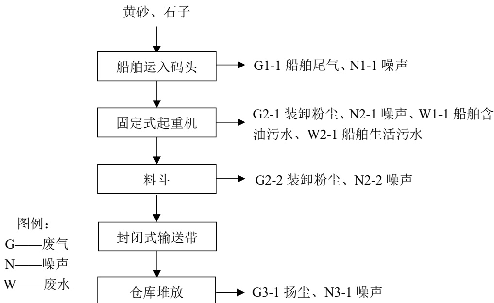
图 4-1 项目工艺流程及产污节点图
